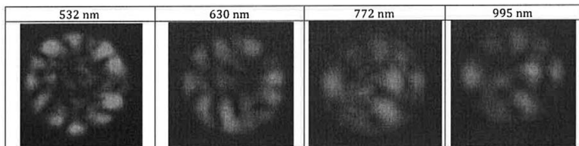
Figure II-36 – De gauche à droite : modes en champ proche en sortie de convertisseur réalisé avec un capillaire Polymicro de 50 µm de diamètre de cœur rempli de DMSO, à 532 nm (énergie incidente de 0,1 µJ), à 630 nm (énergie incidente de 0,74 µJ), à 772 nm (énergie incidente de 1,78 µJ) et 995 nm (énergie incidente de 2,9 µJ).
