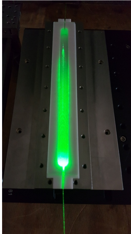
Figure IV-13 – Photo de la cuve en téflon utilisée pour les expériences de diffusion Raman évanescente. La cuve contient une nanofibre de 7 cm de long et de 350 nm de rayon, immergée dans de l'éthanol. Le laser de pompe à 532 nm est injecté via un objectif de microscope (non présent sur la photo) dans l'extrémité situé vers le haut de la photo.
