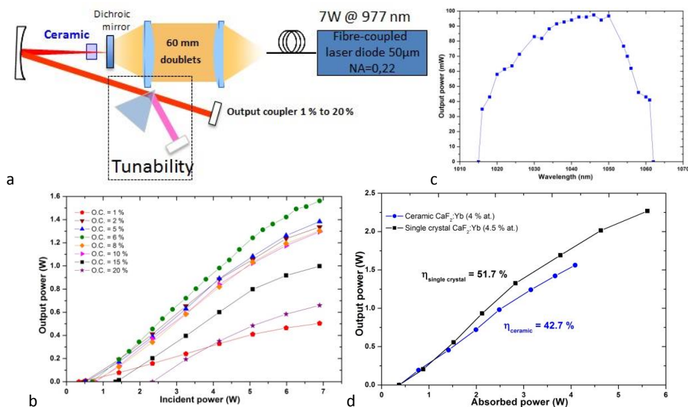
Fig. 1: Résultat laser d'une céramique \text{Yb}:\text{CaF}_2 : dispositif expérimental, puissance de sortie en fonction du coupleur, accordabilité et comparaison avec un monocristal.
