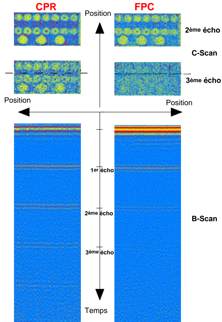
Figure 6. B-scans et C-scans du balayage laser-ultrasons de la plaque de graphite epoxy de la figure 5 obtenus avec un capteur Fabry-Perot confocal de 1 m avec des miroirs de 85 % en mode transmission ainsi qu'avec un capteur photoréfractif basé sur l'InP:Fe sous tension.
